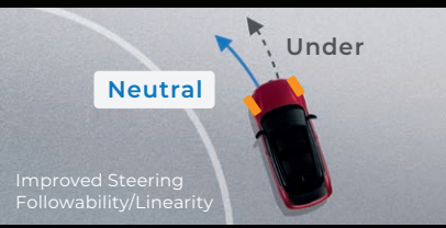
Electric Power Steering-Variable Gear Ratio (VGR) พวงมาลัยพาวเวอร์ไฟฟ้า พร้อมอัตราทดเกียร์แบบแปรผัน
